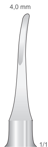
51-130-04 150 mm
