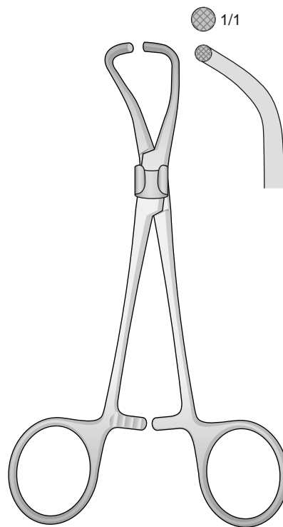
05-590-01 Ø 9 mm 590-03 Ø 12 mm 05-590-02 Ø 14 mm 590-04 Ø 17 mm 130 mm 05-590
