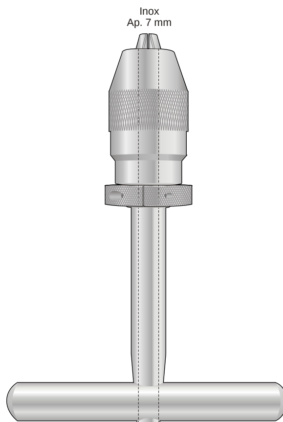
12-1550 135 mm
