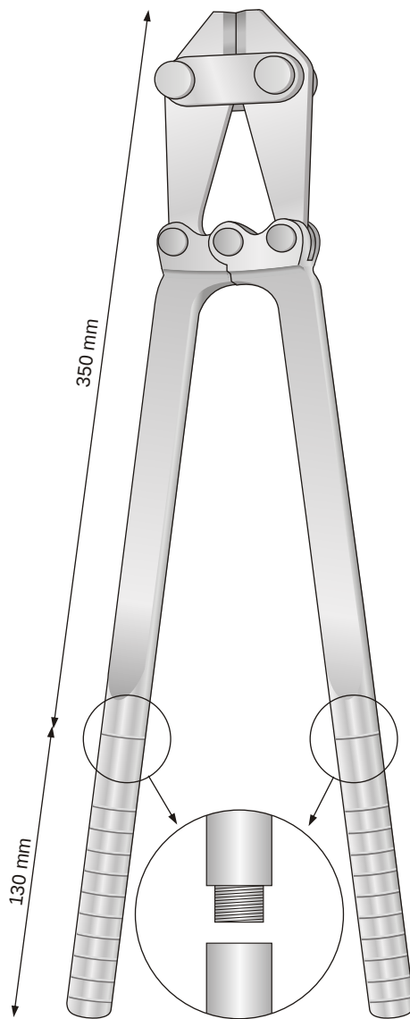
12-1900-02 480 mm
