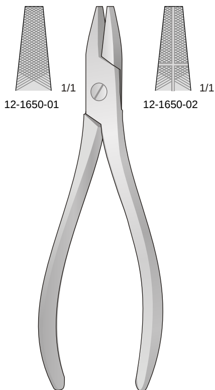
12-1650 175 mm
