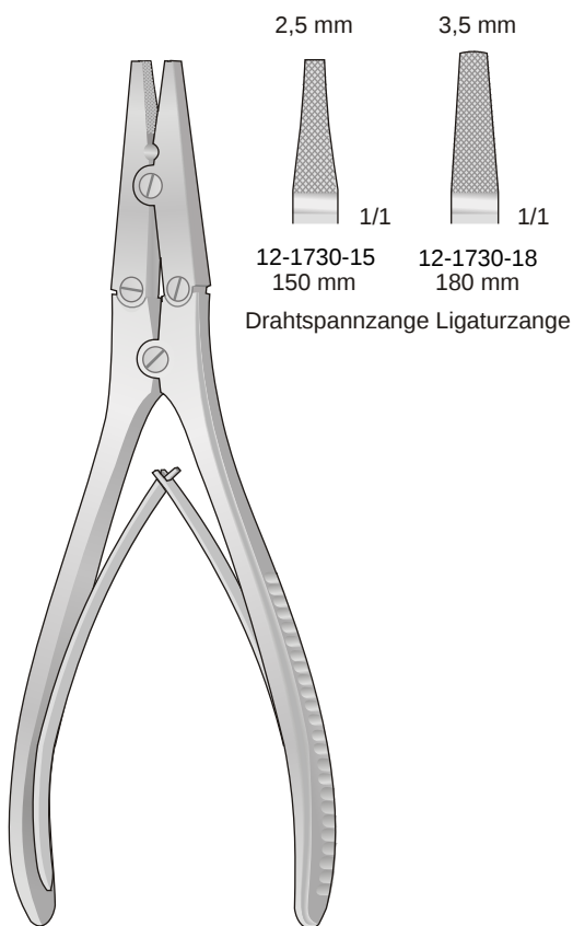
12-1730
