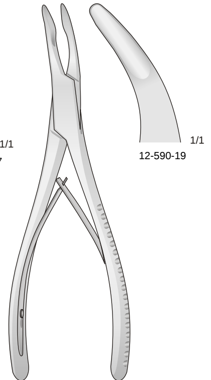
OLIVECROWA 12-590 190 mm
