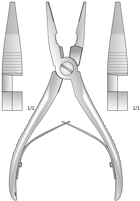
12-1690-17 175 mm
