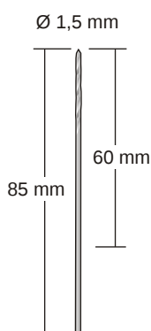
12-1980-02
