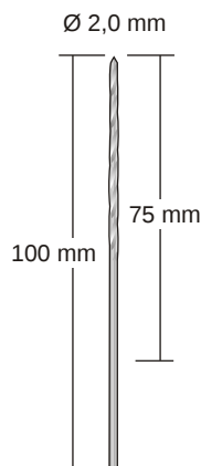
12-1980-03
