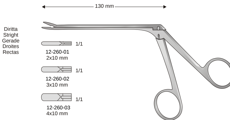
LOVE-GRUENWALD 12-260
