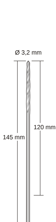
12-1980-06
