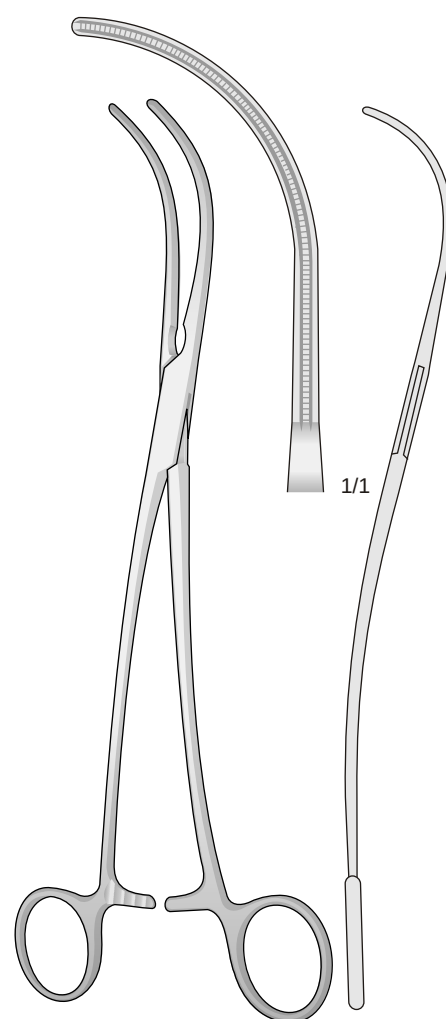
De BAKEY 06-950-24 240 mm
