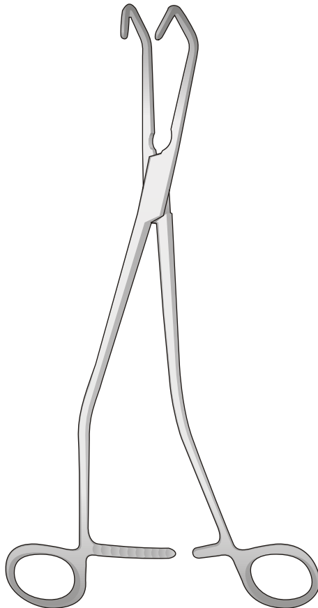
HOPT 06-1480-01 - 230 mm 06-1480-02 - 235 mm 06-1480-03 - 240 mm
