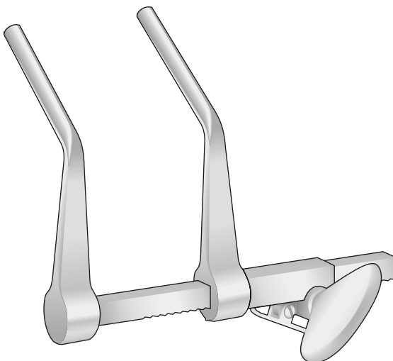
CASPAR 18-2840-02 Distraktor links, Allein Distractor left, Only Distrattore sinistro, solo
